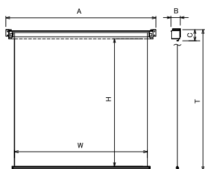
■外形寸法図
