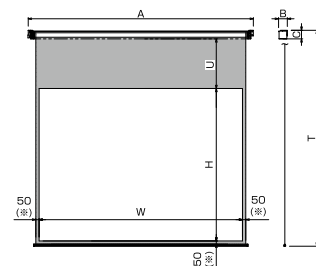
■外形寸法図
