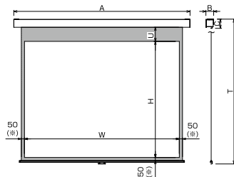
■外形寸法図
